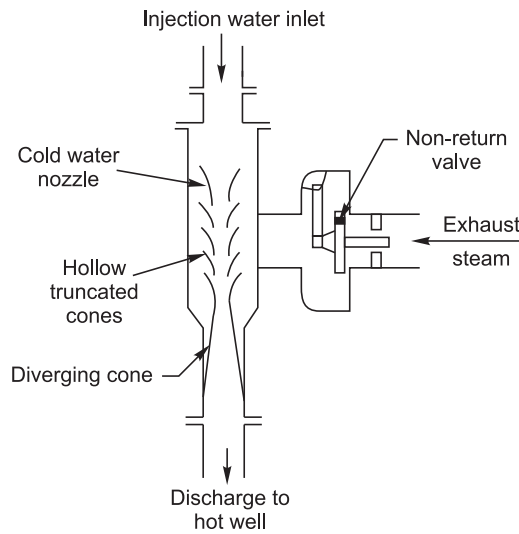
Fig. 1.22. Ejector Condenser
